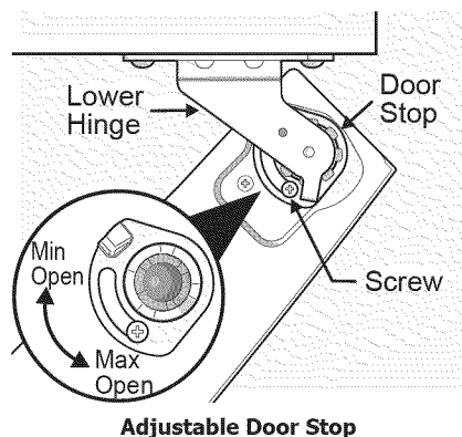
Adjustable Door Stop
